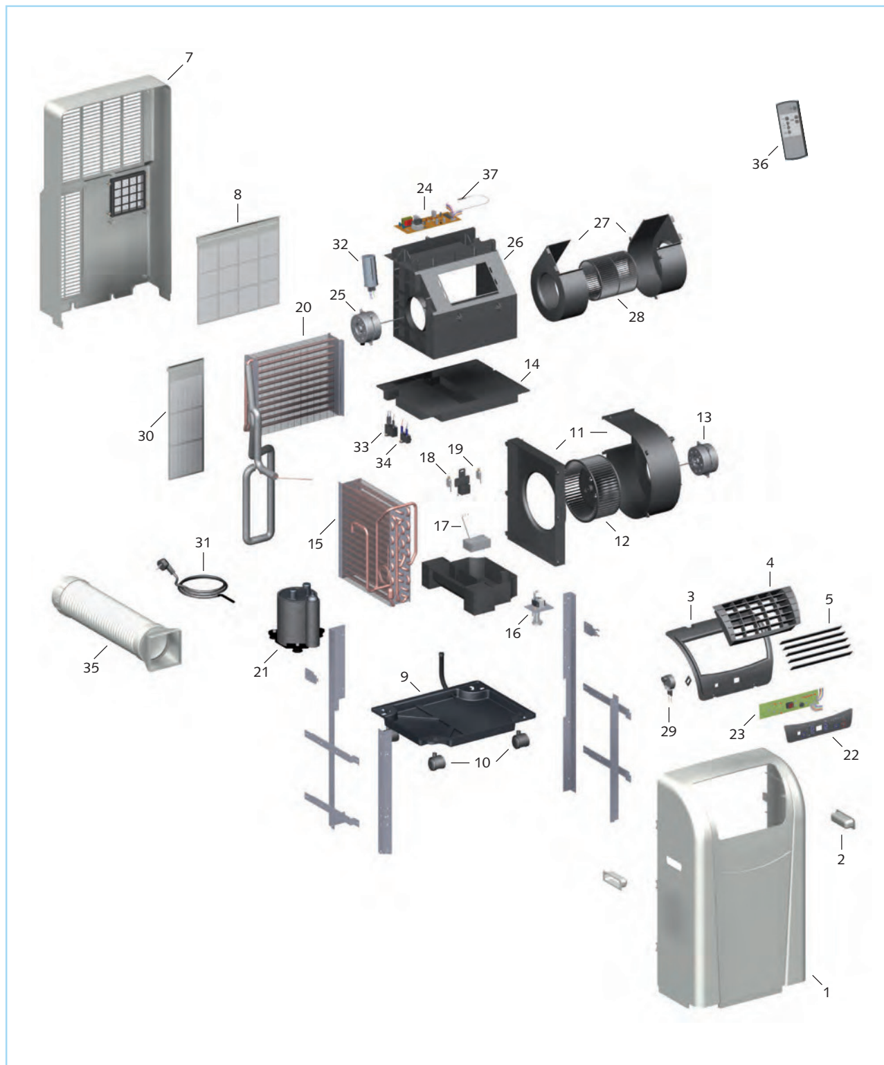
Abb. 18: Explosionszeichnung
