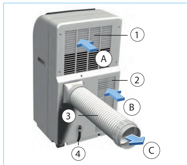
Abb. 2: Rückansicht
